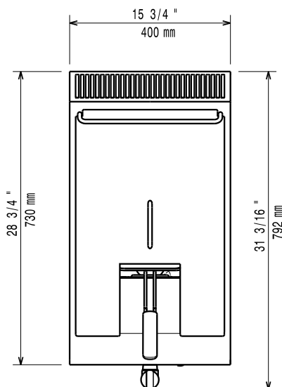
Boven aanzicht
